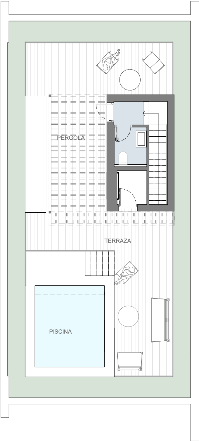
PLANTA CUBIERTA
