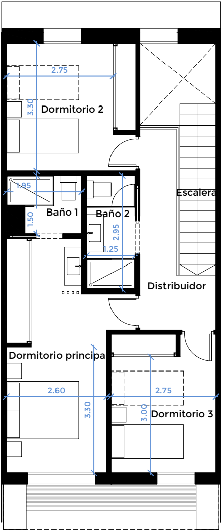
PLANTA PRIMERA
