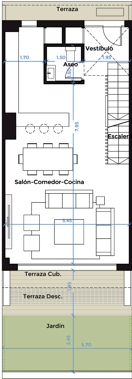
PLANTA BAJA
