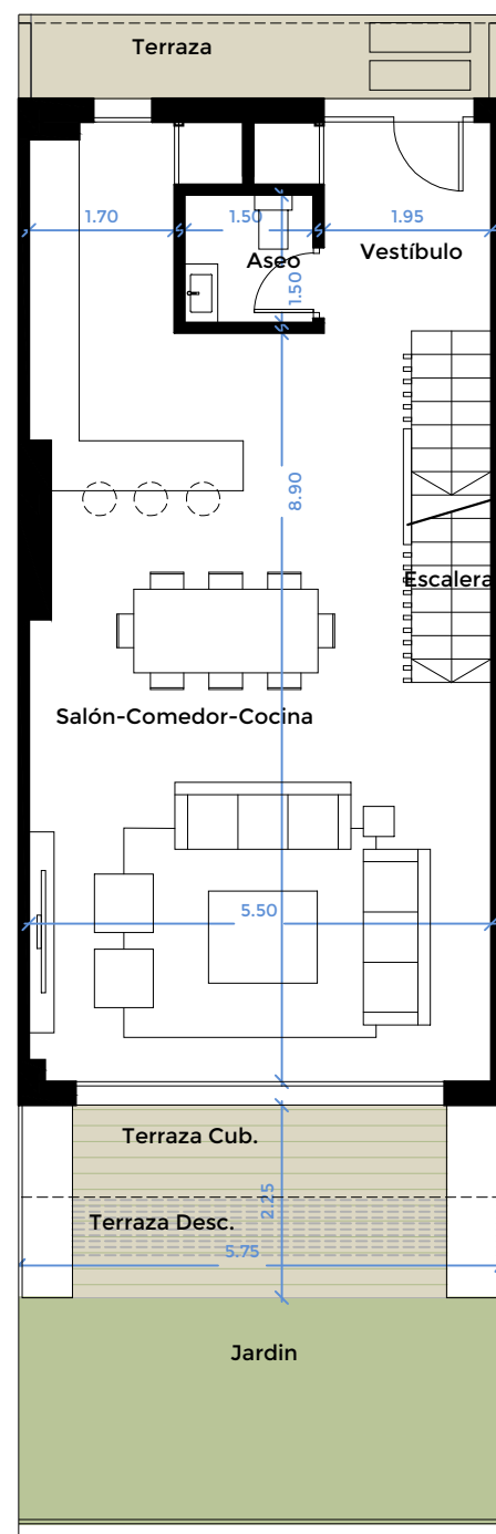
PLANTA BAJA
