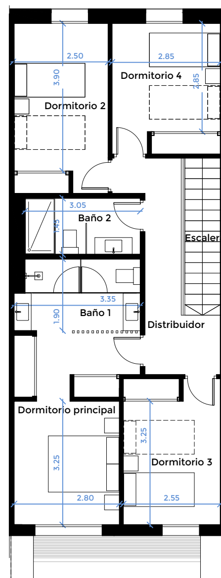
PLANTA PRIMERA
