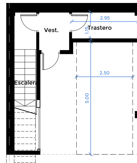
PLANTA SÓTANO
