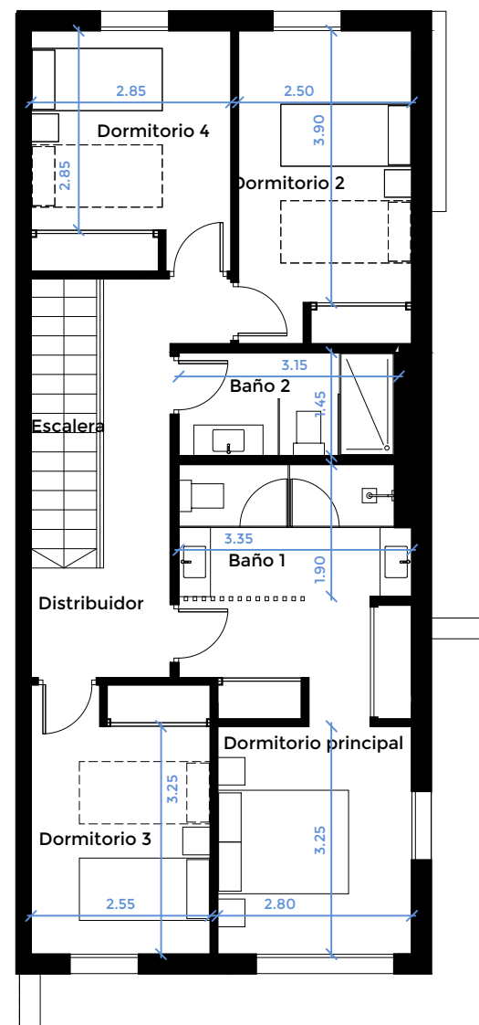
PLANTA PRIMERA
