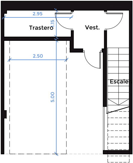
PLANTA SÓTANO
