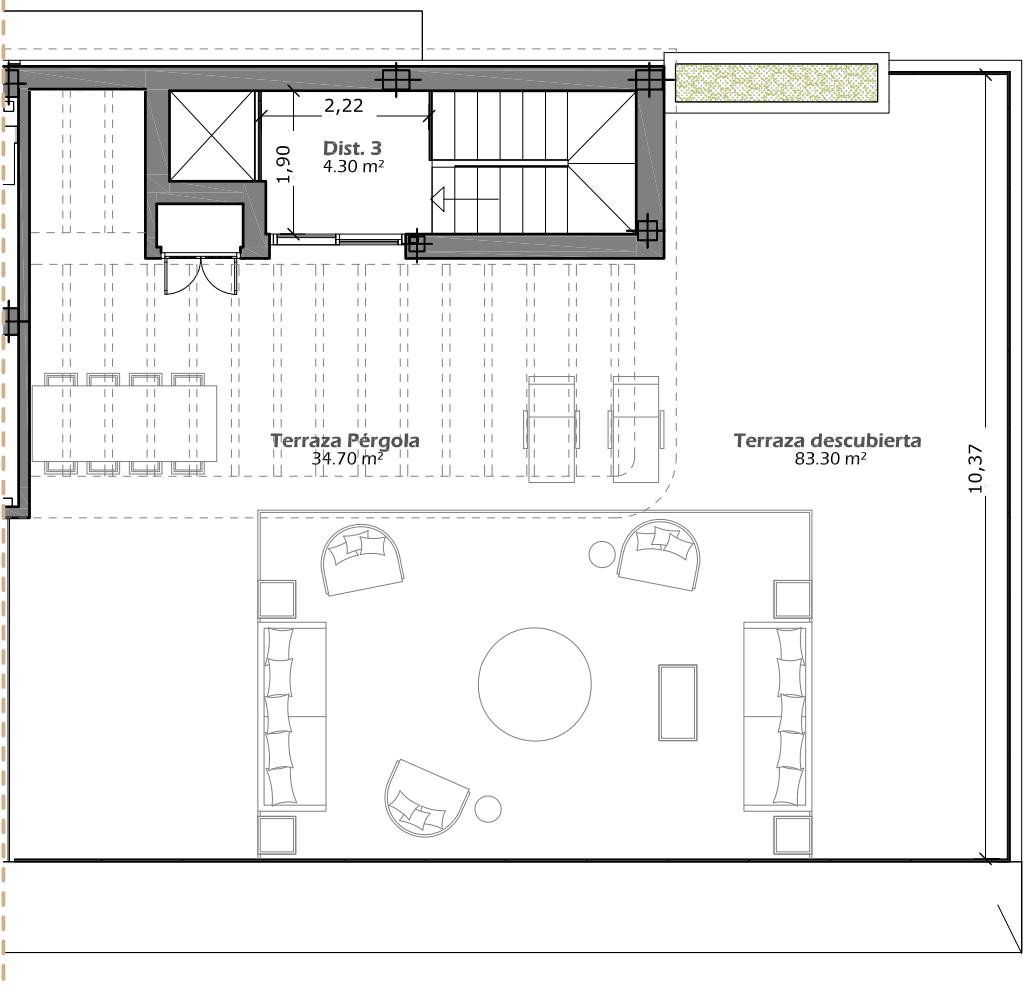
Planta Solarium
