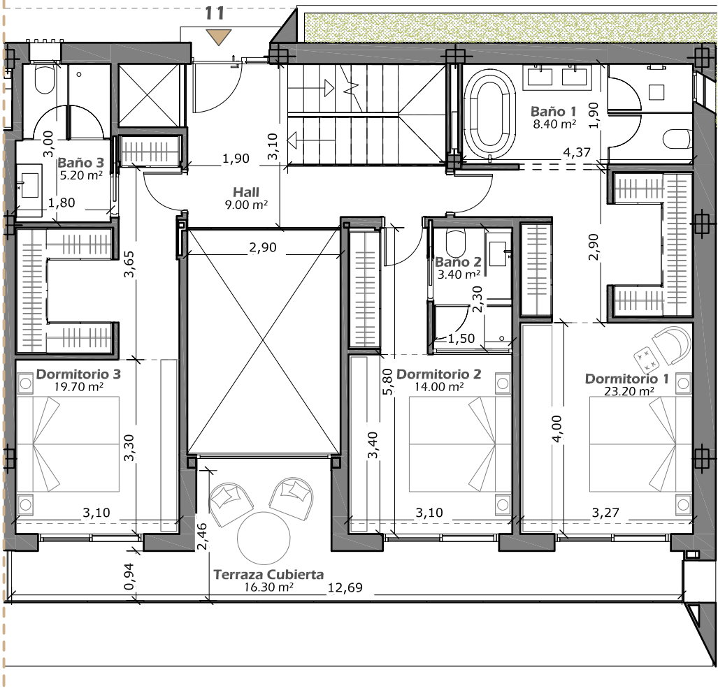
Planta Primera
