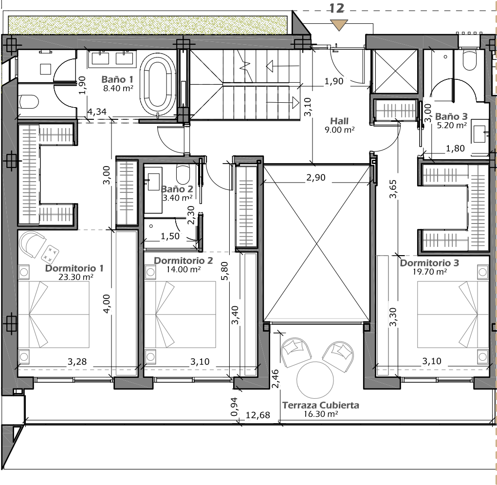
Planta Primera
