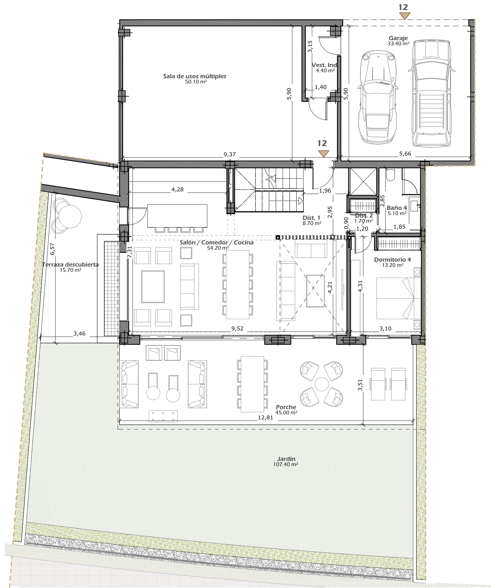
Planta Baja
