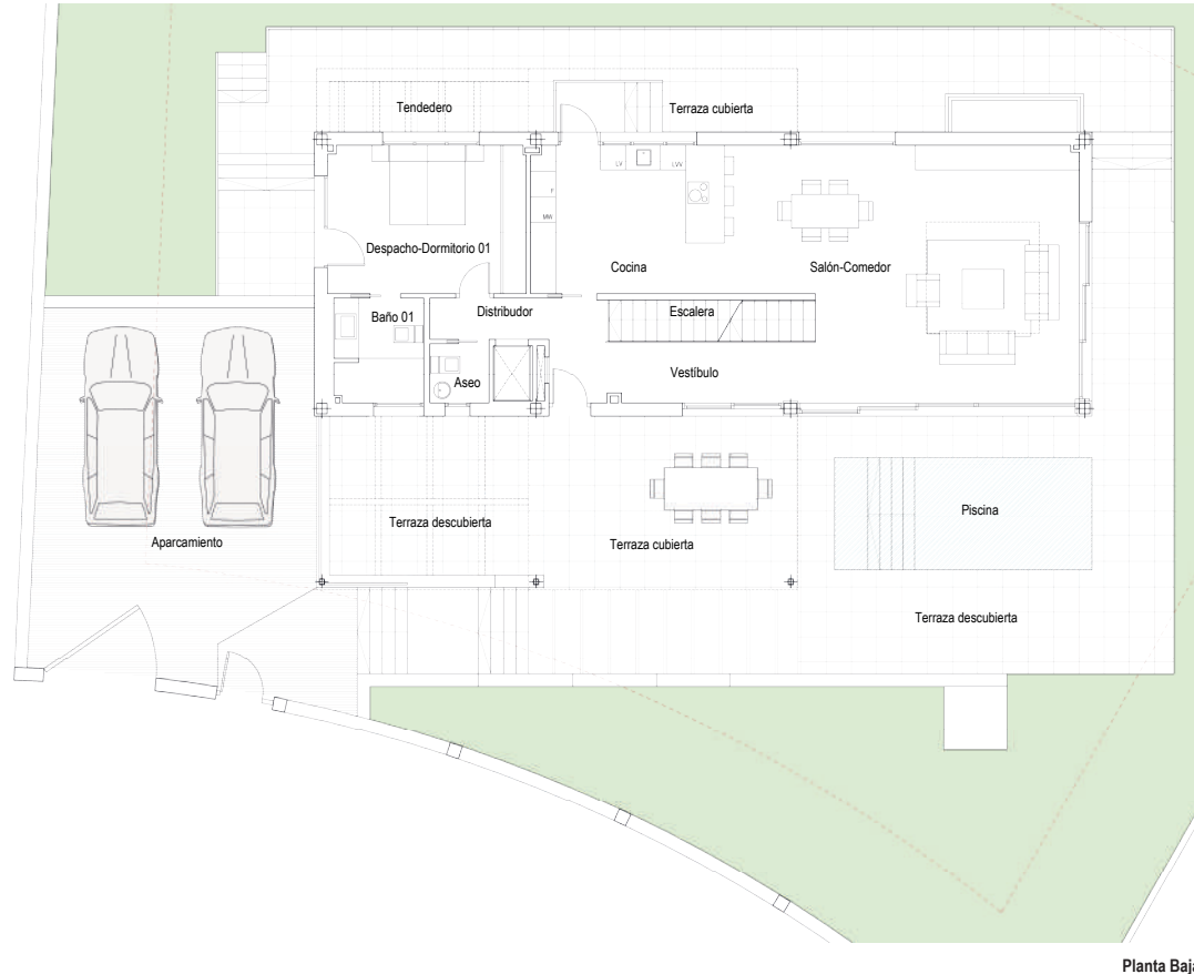
Planta Baja
