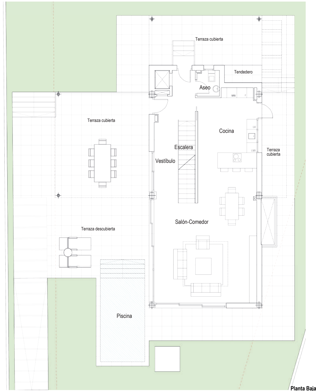
Planta Baja
